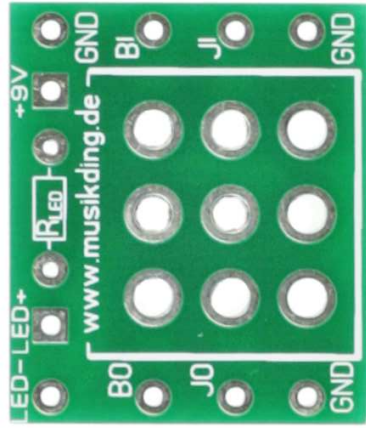
Top Side Oberseite
