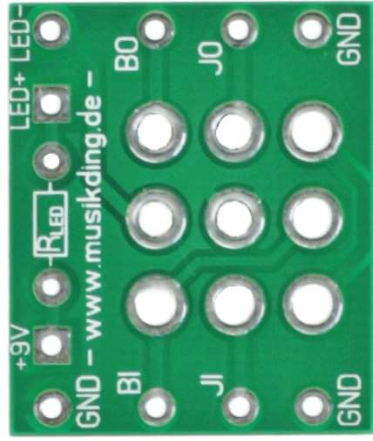
Bottom Side Unterseite
